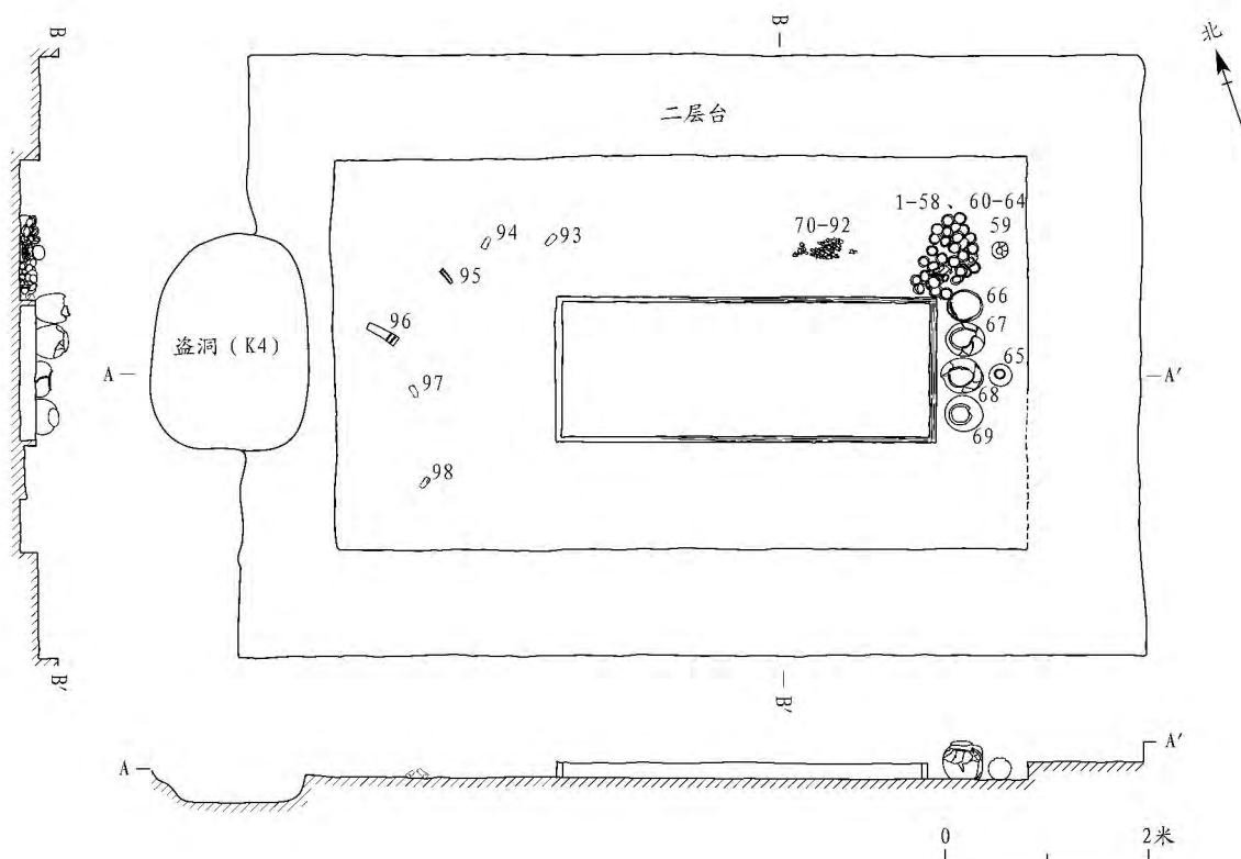
图三// 马脊墩M1平面图、剖视图
