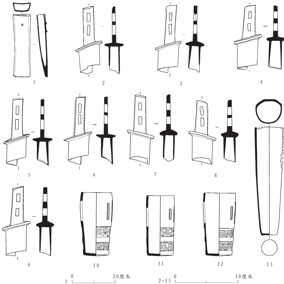
图七// 马脊墩M1出土铜饰件及铜车器
