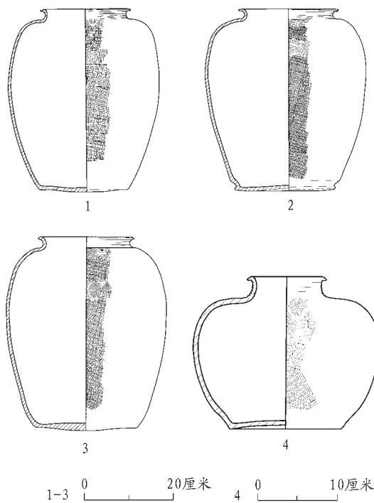
图六// 马脊墩M1出土硬陶器
