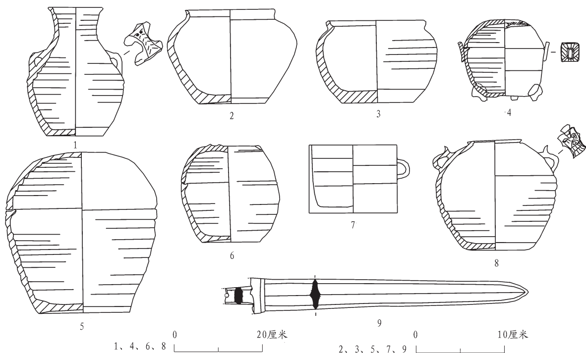
图六// M9出土器物
