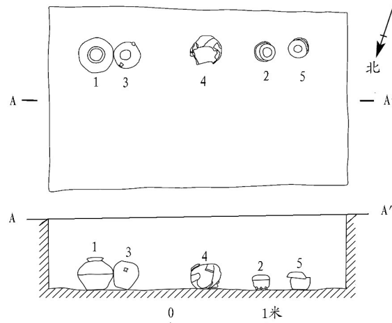
图七// M10平、剖面图
