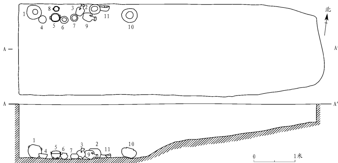
图一—// M8平、剖面图
