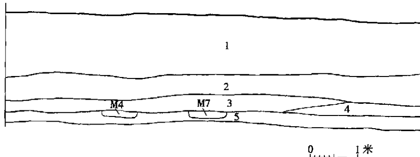
图三 B 区 T1 北壁剖面图
