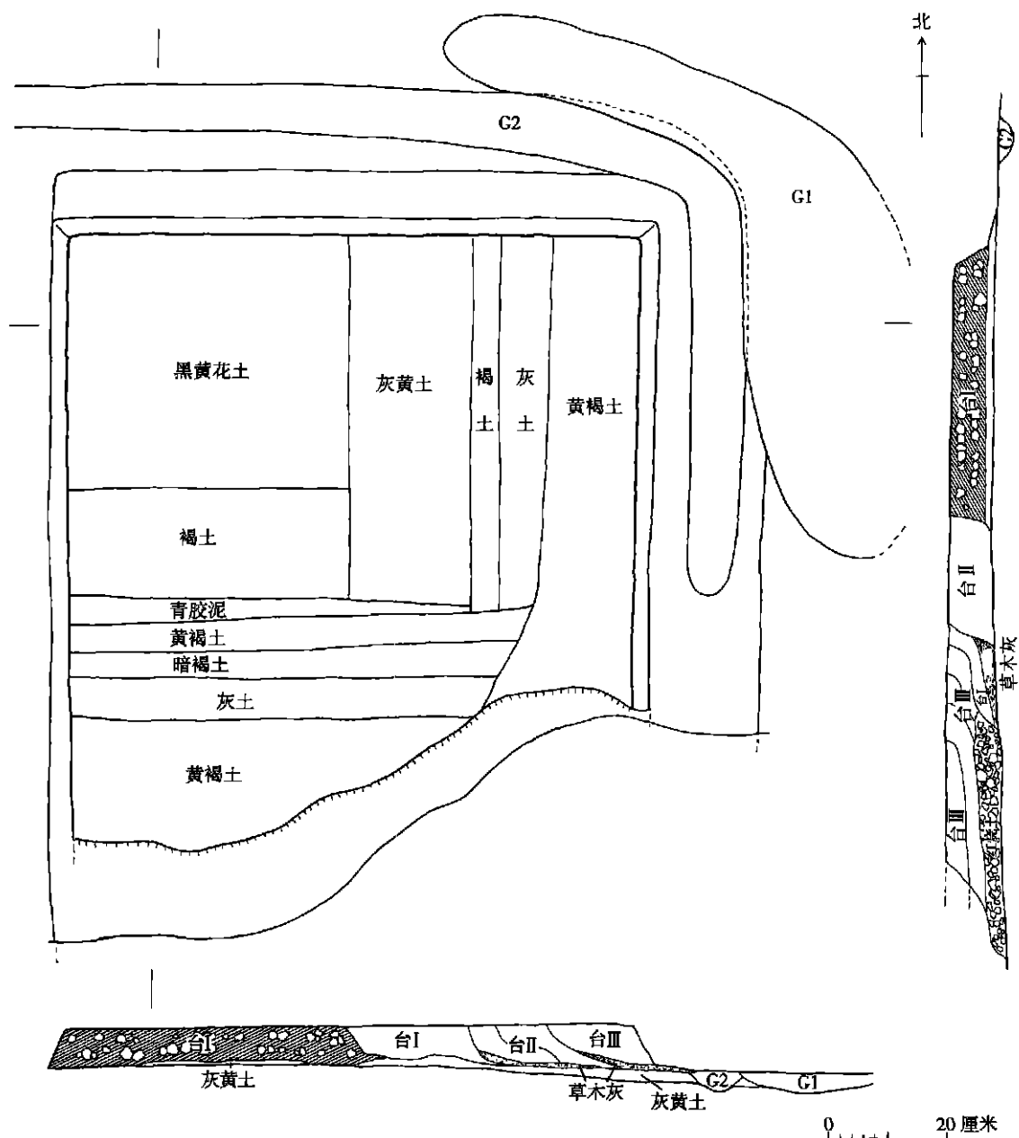
图五 祭台平、剖面图
