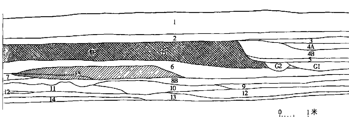
图二 A区 T401 北壁剖面图
